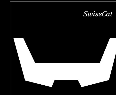
Querschnitt SwissCat-Rumpf.
